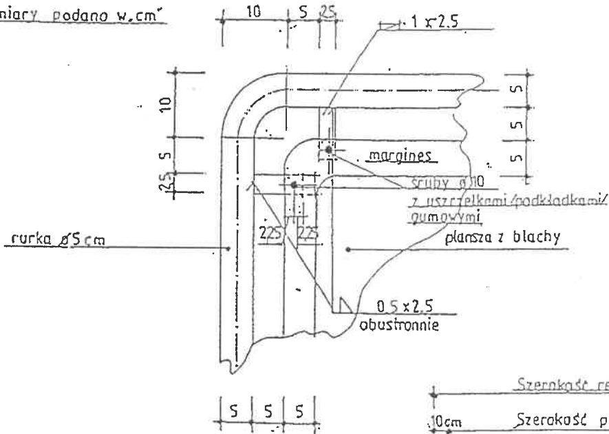
SZCZEGÓL: KONSTRUKCYJNY "A"
